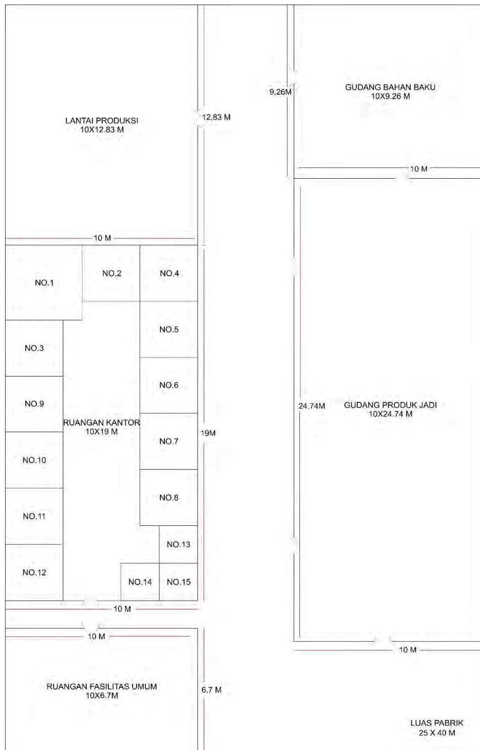
Gambar 2. Layout Pabrik
