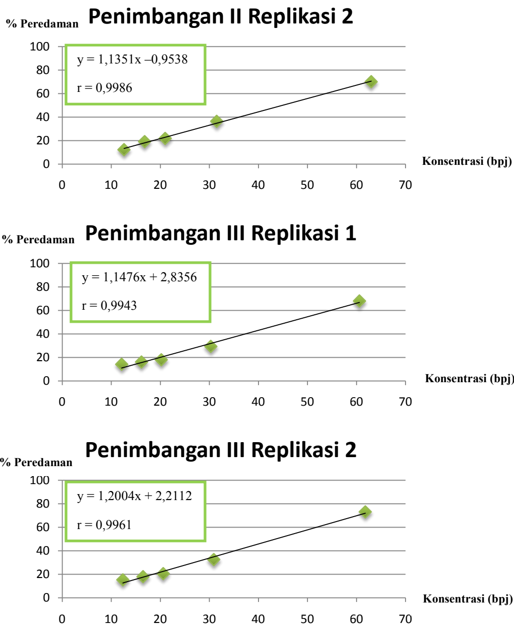
Gambar 8 Kurva Konsentrasi Ekstrak Etanol Kulit Buah Manggis Freeze Drying vs % Peredaman Radikal Bebas DPPH Penimbangan II Replikasi 2, Penimbangan III Replikasi 1 dan 2.
